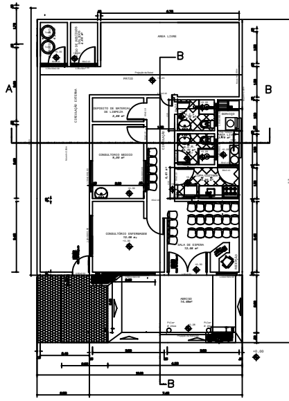
PLANTA BAIXA ESCALA 1/75
